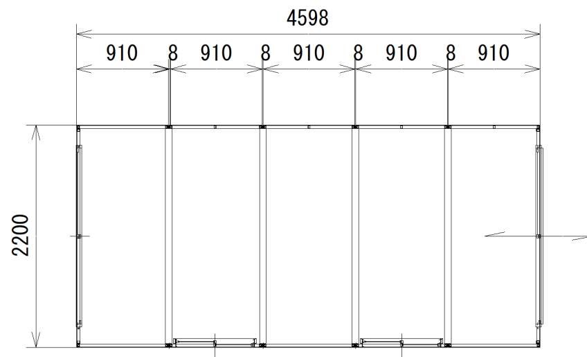
平面図 S=1:50
