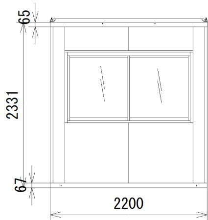
D立面図 S=1:50
