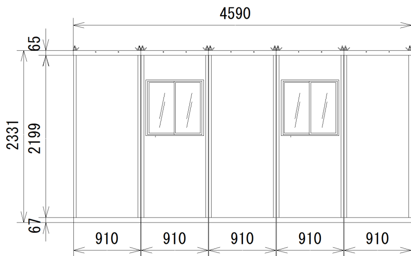
C立面図 S=1:50
