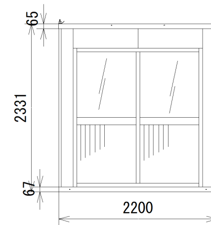
B立面図 S=1:50
