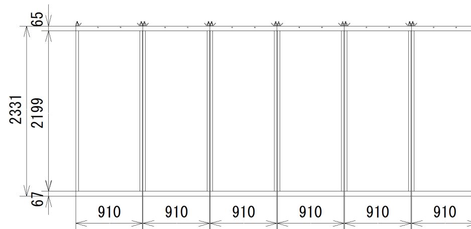
A立面図 S=1:50
