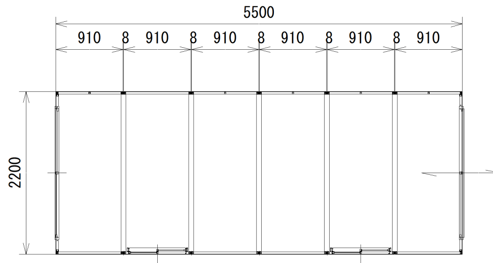
平面図 S=1:50
