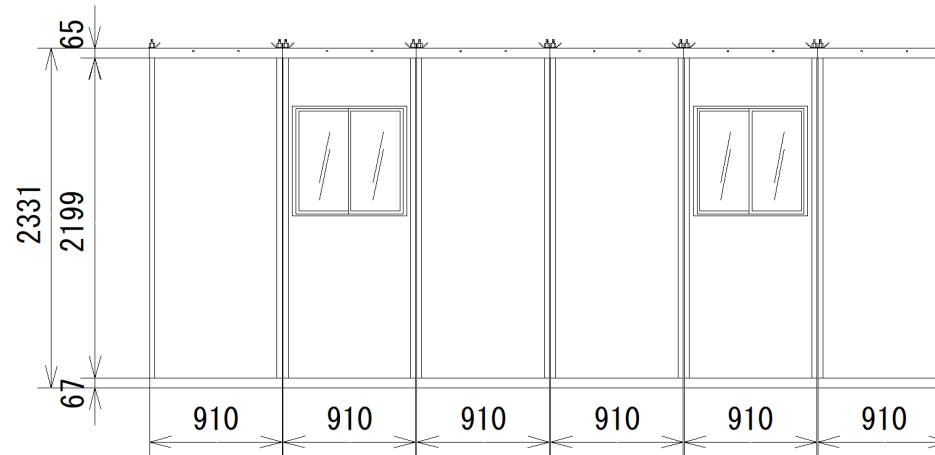
C立面図 S=1:50
